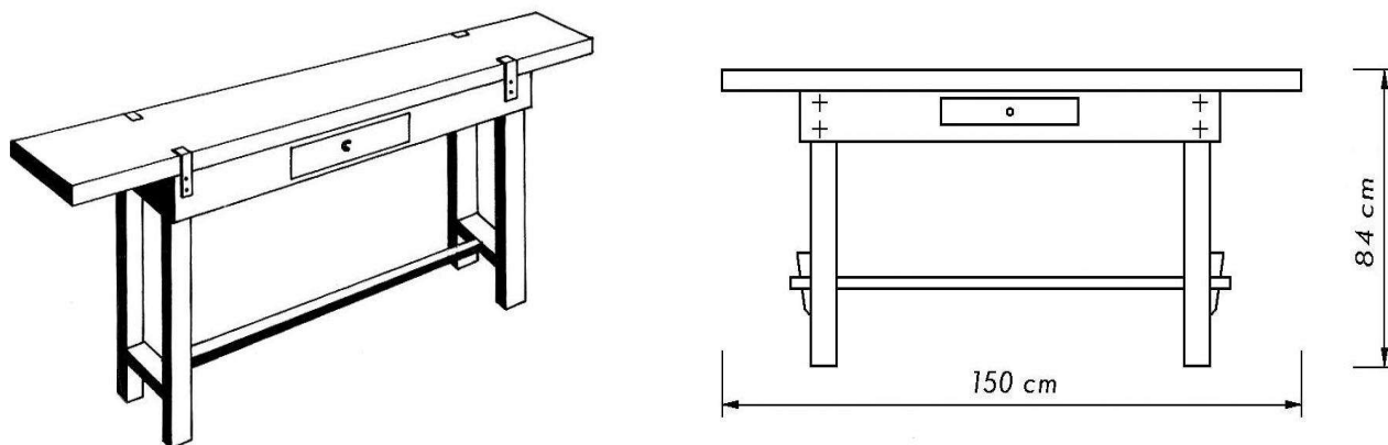
Fig. 193 – Bancada de trabalho (modelo D.G.A.C.)
